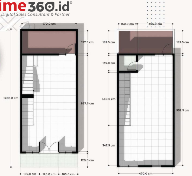
Lantai Dasar
