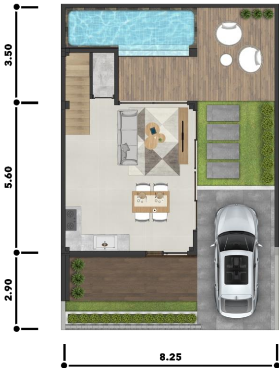
FLOOR PLAN TAHAP 1
